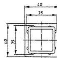
Verschlusskappe für 40mm Schiene
