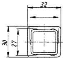
Verschlusskappe für 30mm Schiene
