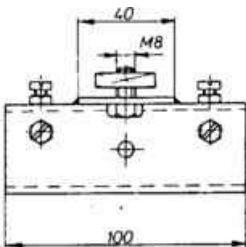
Schienenhalter- und Verbinder für 30mm Schiene
