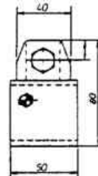
Schienenhalter mit 4-kant Mutter für 40mm Schiene
