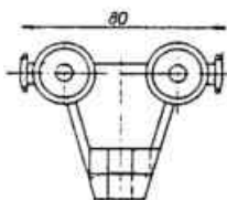
Leitungswagenoberteil für 30mm Schiene
