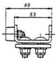
Endanschlag für 30mm Schiene
