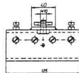
Schienenhalter- und Verbinder für 40mm Schiene
