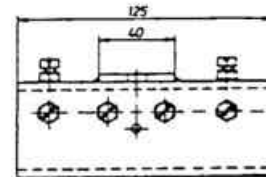
Schienenhalter- und Verbinder für 40mm Schiene
