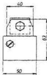
Schienenhalter mit 4-kant Mutter für 30mm Schiene
